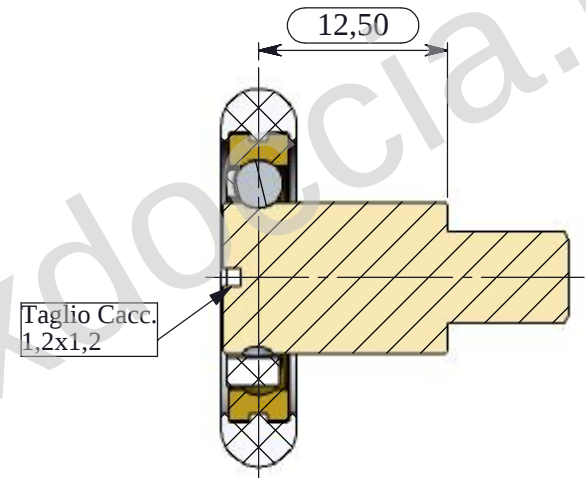
SEZIONE A-A SCALA 2 : 1
