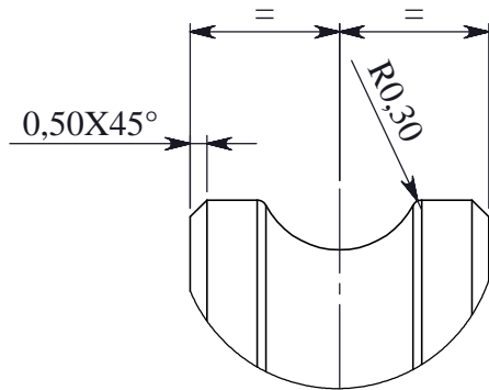
DETTAGLIO B SCALA 4 : 1
