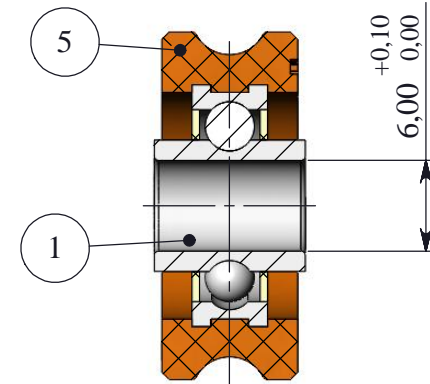
SEZIONE A-A SCALA 2 : 1
