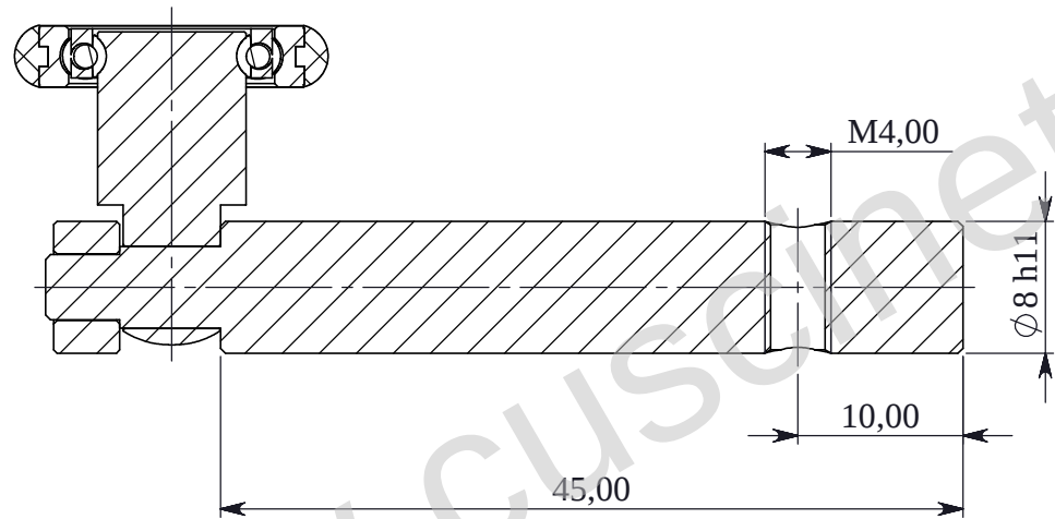
SEZIONE A-A
