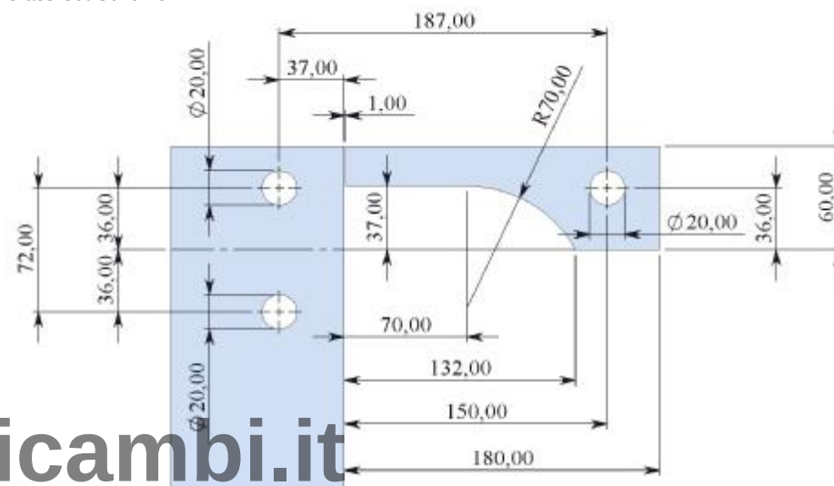
Schema per Taglio Vetro Glass Cut Scheme
