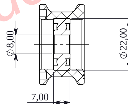
SEZIONE B-B SCALA 1 : 1
