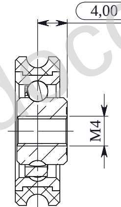
SEZIONE A-A
