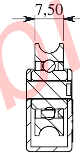
SEZIONE A-A
