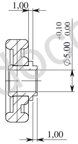
SEZIONE A-A
