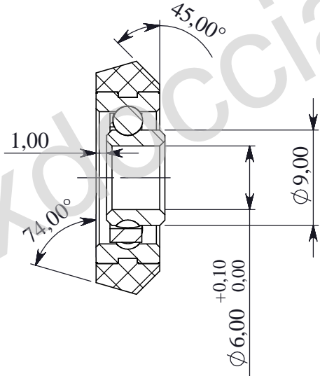
SEZIONE A-A
