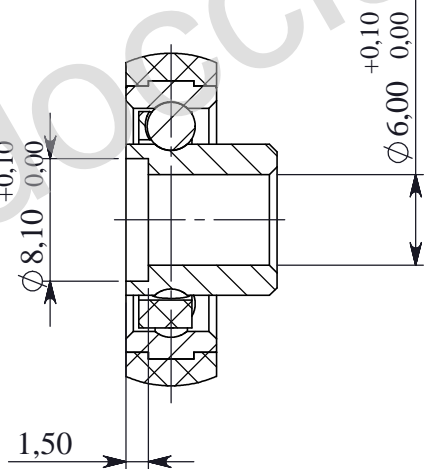
SEZIONE A-A
