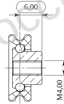
SEZIONE A-A
