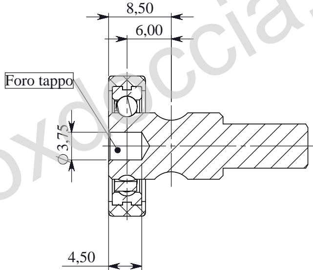
SEZIONE A-A
